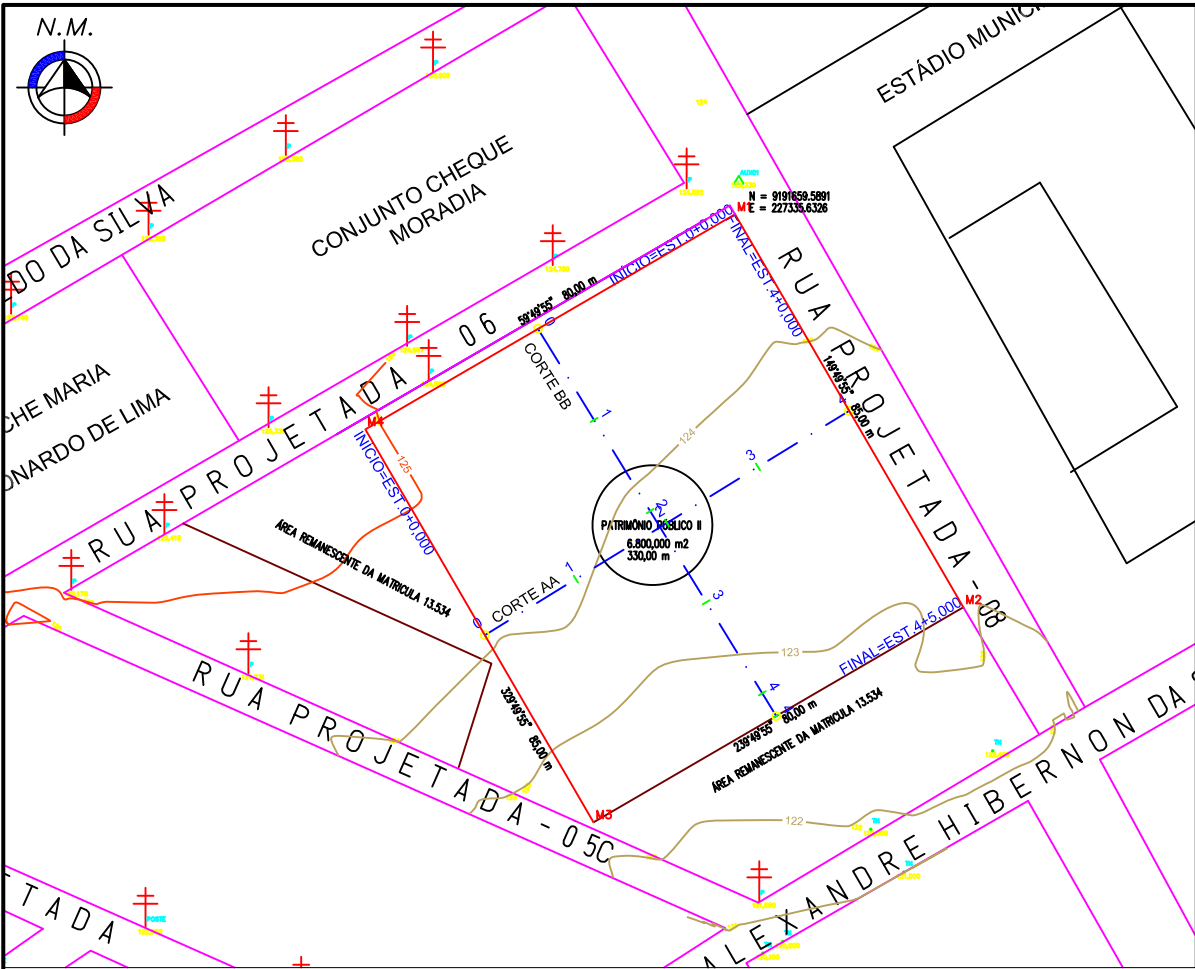
PLANIALTIMÉTRICO ESCALA === 1/1000
